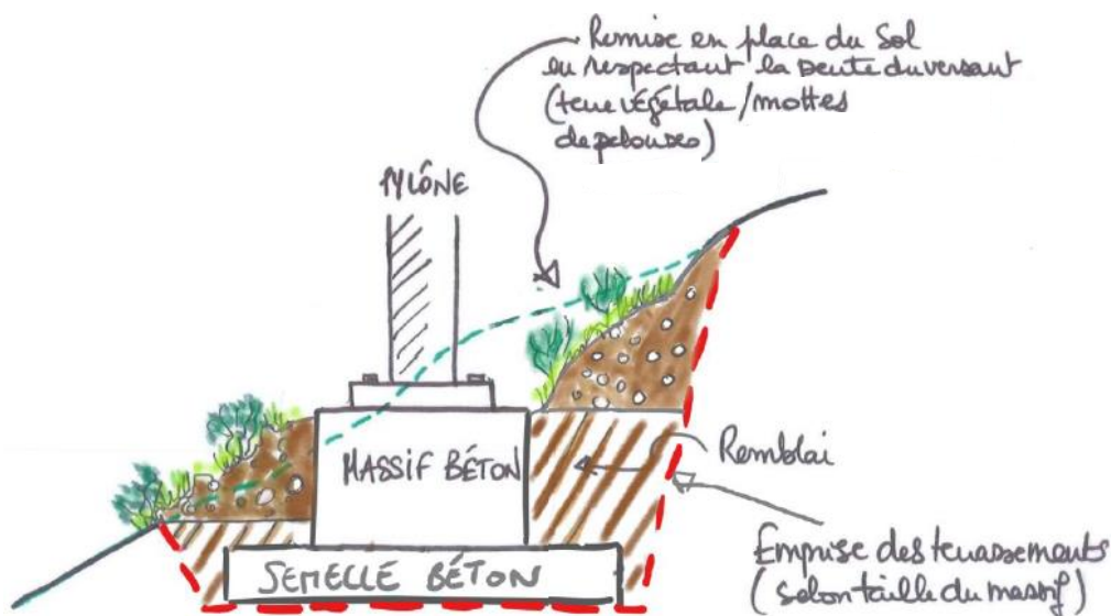
Schéma de principe pour le traitement des emprises de pylônes
