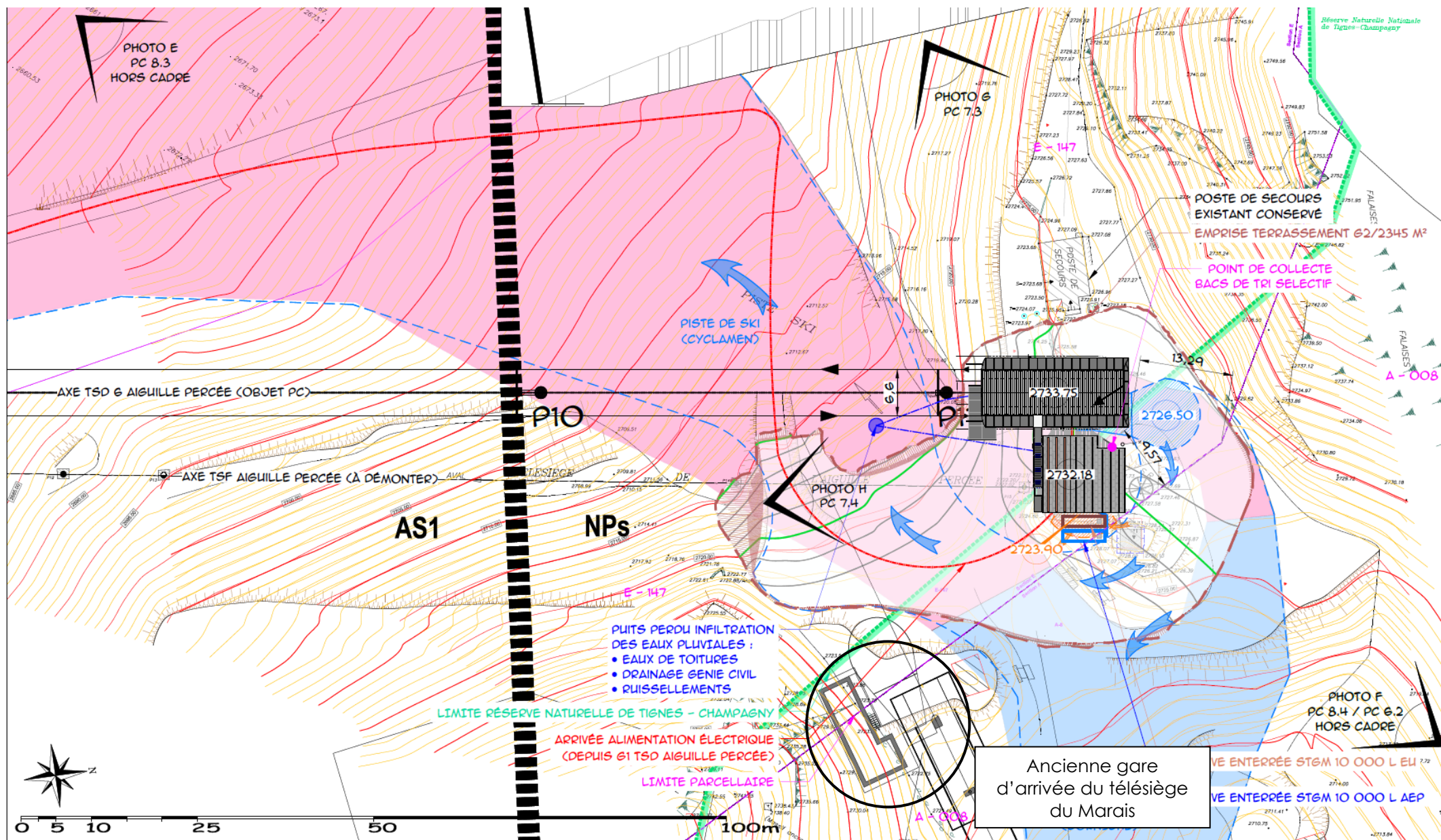
Plan de masse des aménagements de la gare amont (G2) du télésiège de l'Aiguille Percée et localisation de la limite de la réserve naturelle de Tignes Champagny en vert. Source : DCSA.
