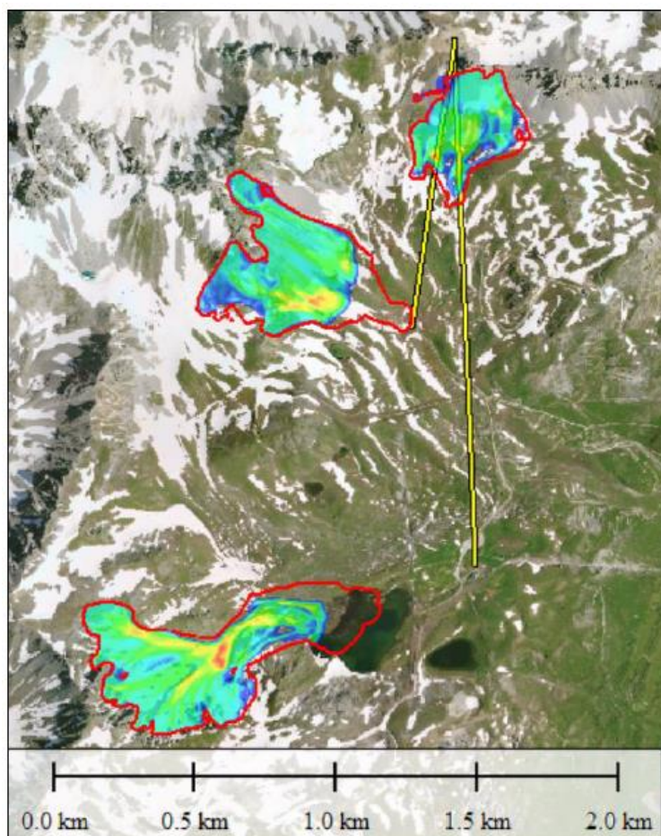
Épaisseur maximale obtenue pour les avalanches denses trentennales. En rouge, limite des avalanches centennales. Source : Diagnostic des risques nivologiques, Engenireesk.
