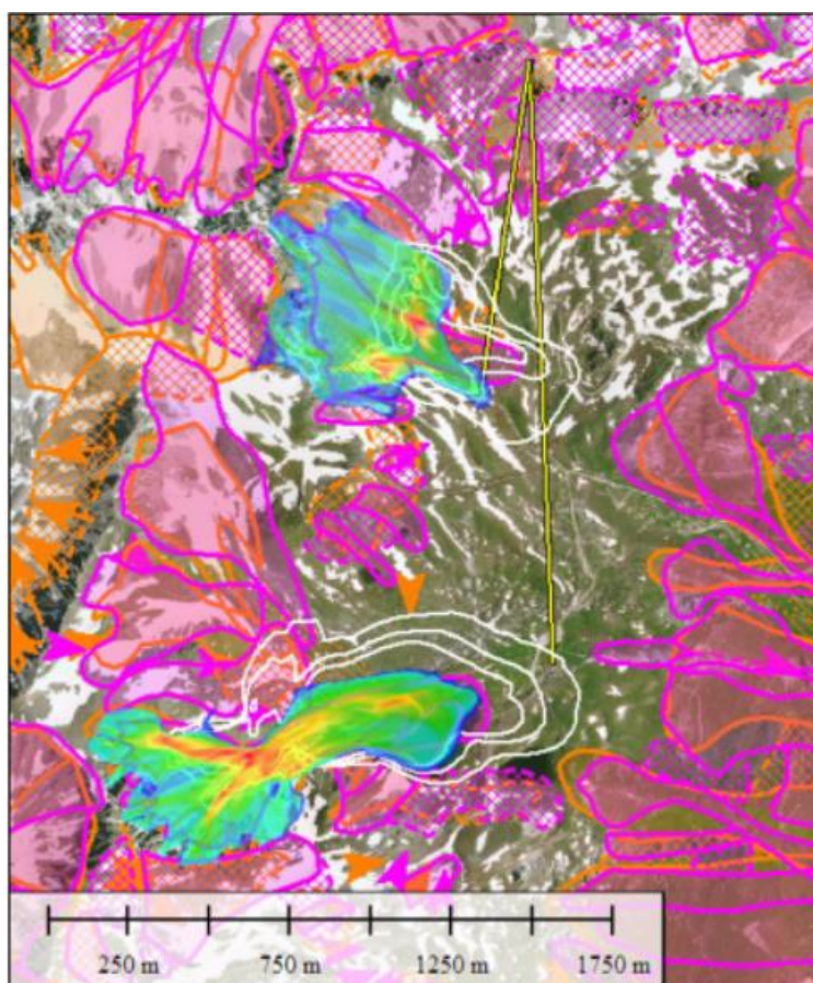
Épaisseur maximale du cœur de l'aérosol (période de retour tri-centennale) et isocontours de la pression du nuage (en blanc). Source : Diagnostic des risque nivologiques, Engineerisk.
