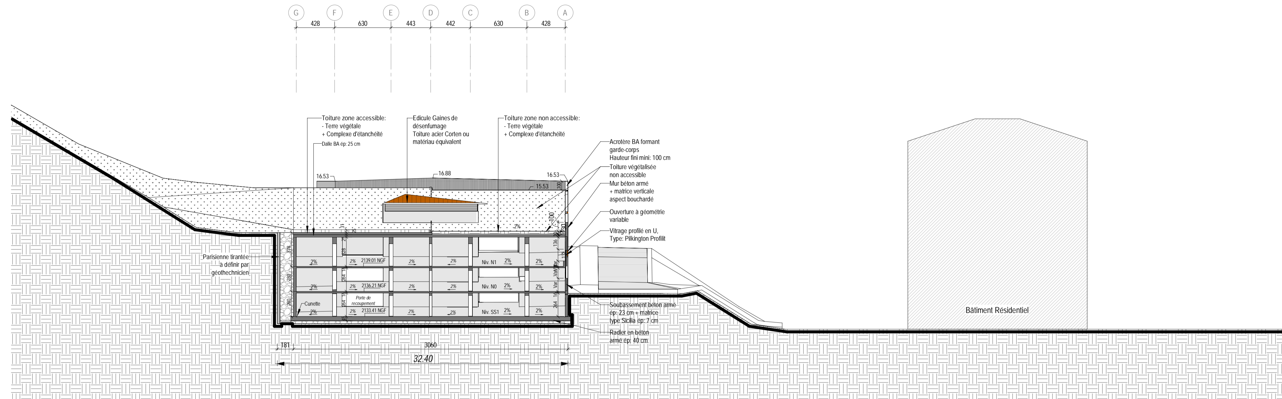
COUPE TRANSVERSALE AA - EST / OUEST FILE C/D SUR PARC DE STATIONNEMENT
