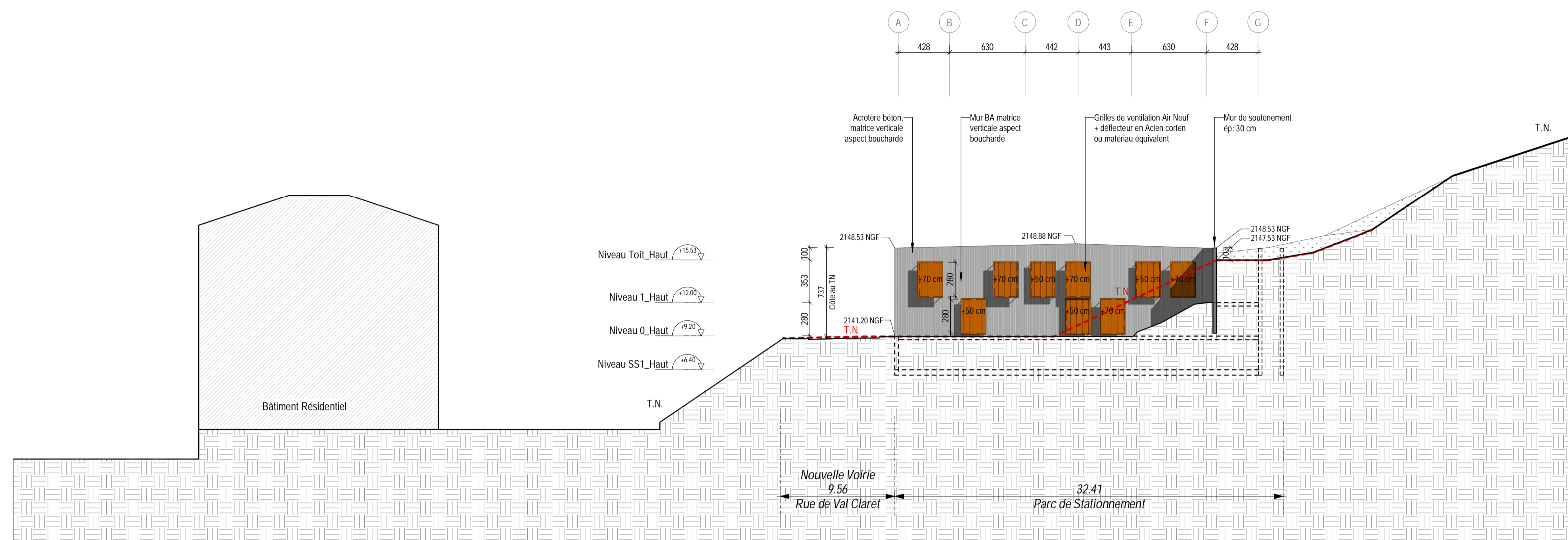
ELEVATION DE LA FACADE PIGNON SUD
