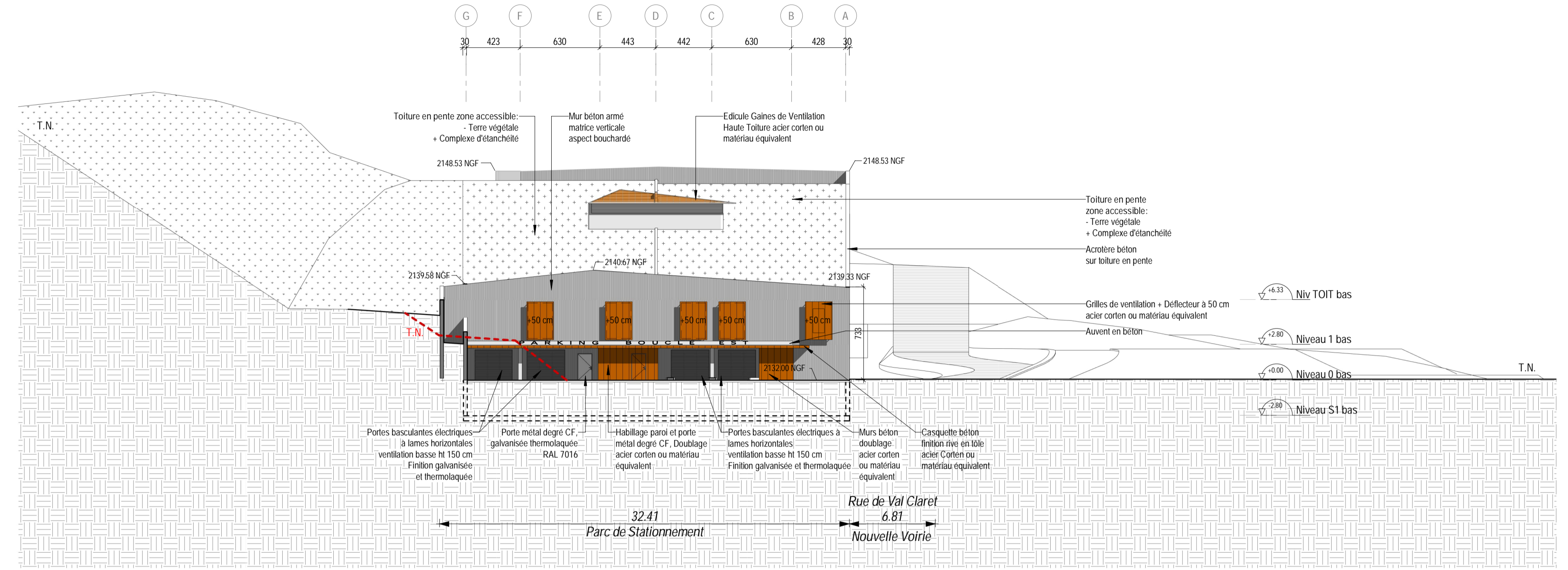
ELEVATION DE LA FACADE PIGNON NORD SUR PLAN D'ACCES
