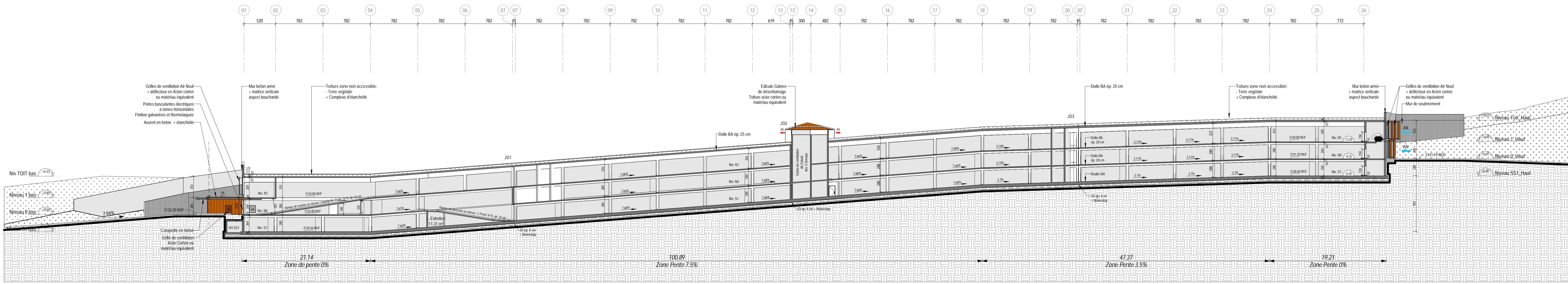
COUPE LONGITUDINALE BB - NORD / SUD SUR PARC DE STATIONNEMENT
